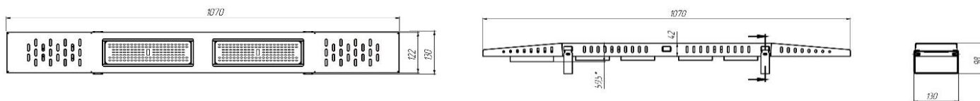
Малюнок 1.2. Габаритні розміри світильника
