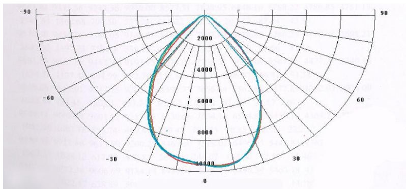
Малюнок 1.1. Крива розподілу сили світла
